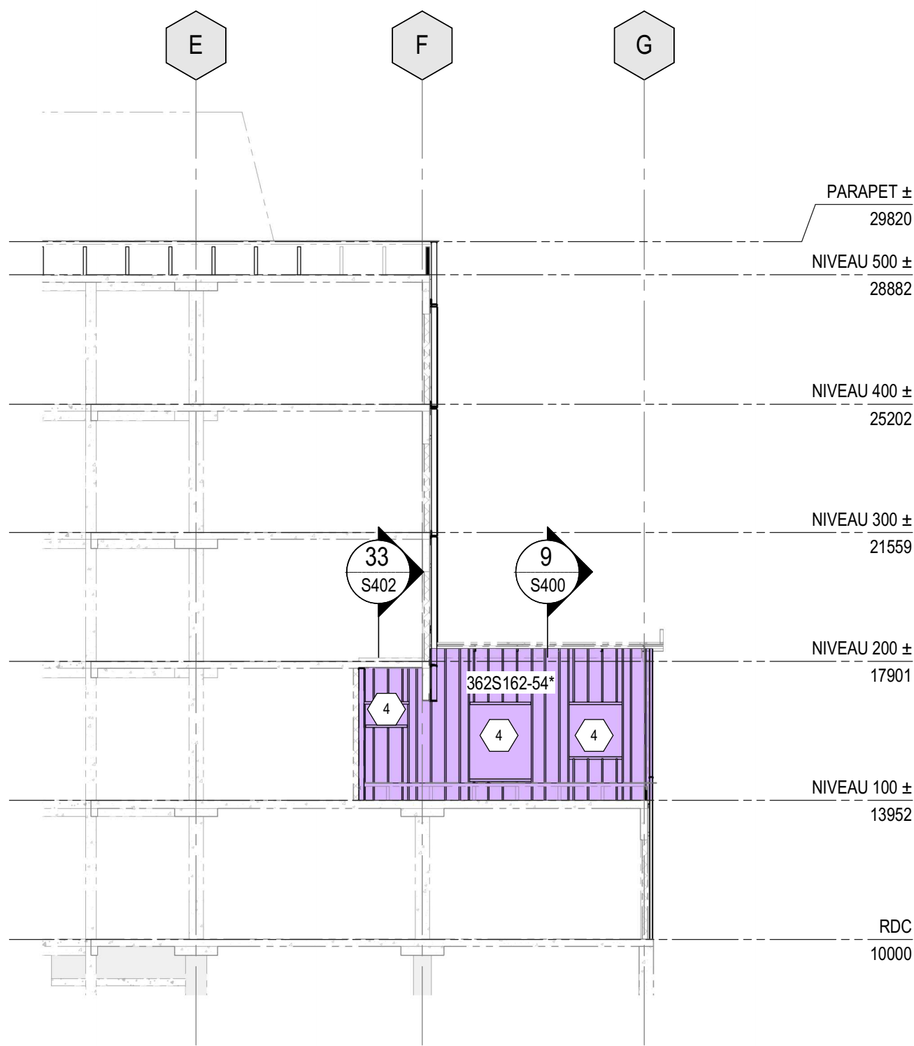
C ÉLEVATION OUEST PARTIELLE S200 1:150
