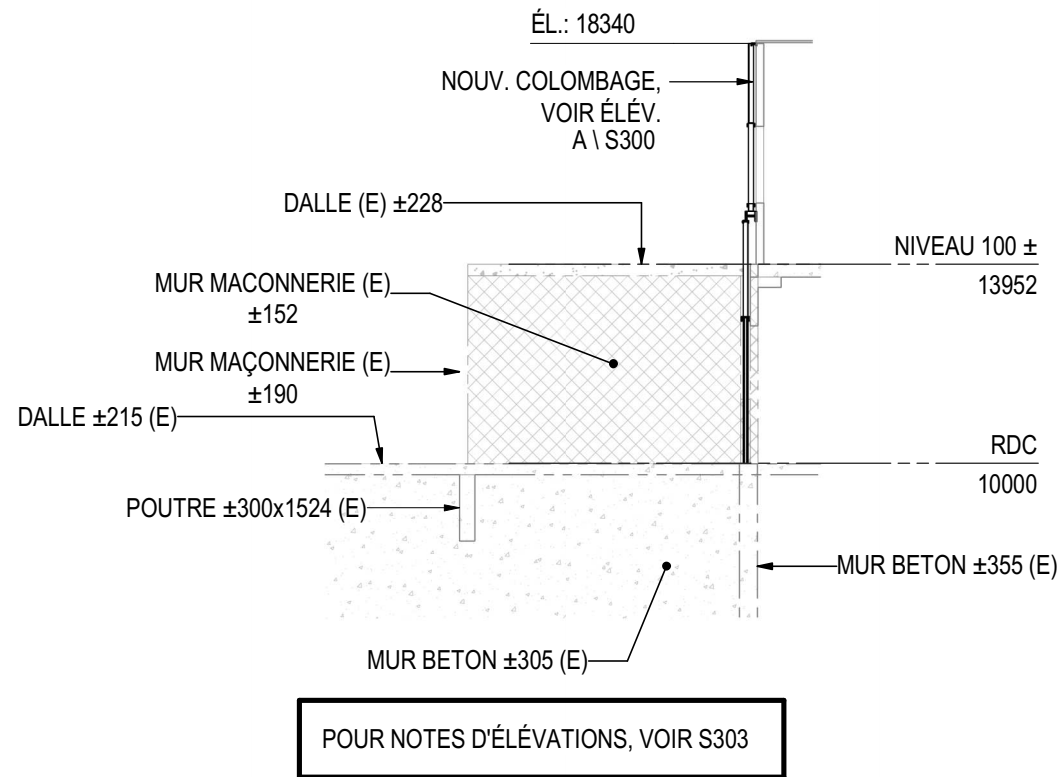
D ÉLEVATION EST PARTIELLE S200 1:150
