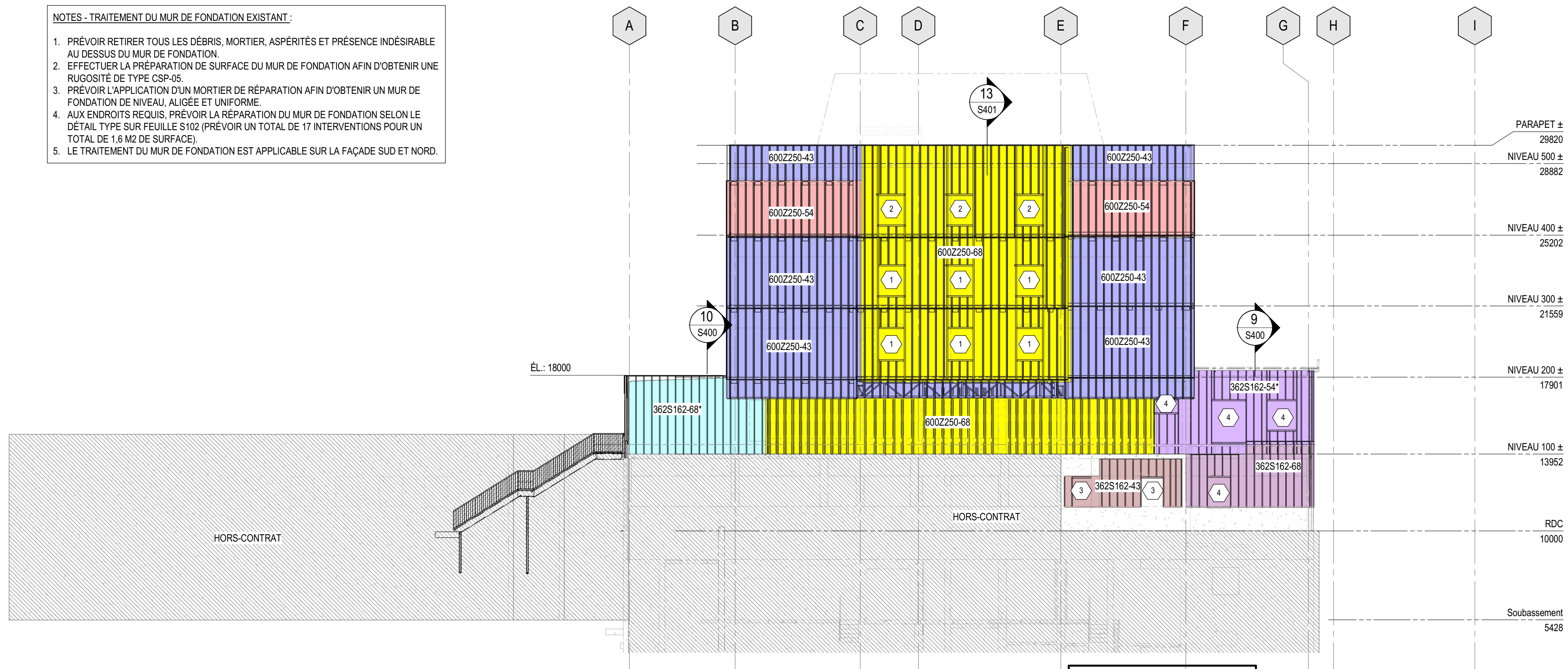
B S200 1:150 ÉLEVATION OUEST
