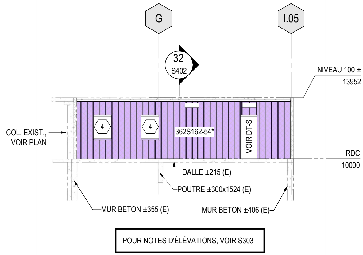
C ÉLEVATION OUEST PARTIELLE S200 1:150
